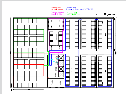
Planung für 410 Sauen inkl. Futtertechnik etc.
